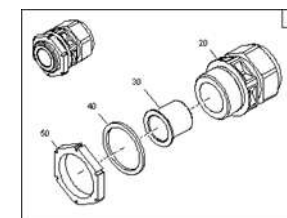
ЕТВ-0000009479, Держатель датчика
