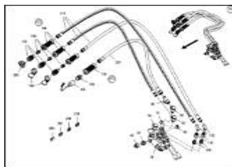
ETV-0000006549, Гидравлический регулирующий клапан в сборе
