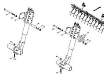
ETB-0000001070, Выравниватель Exakt 1200-2T монтажные детали
