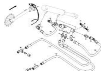
ЕТВ-0000001369, Колесо с почвозацепами гидравлические детали
