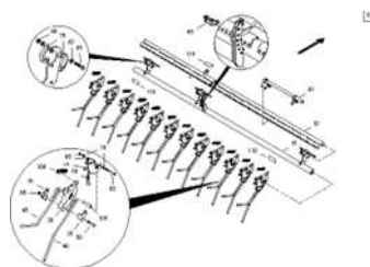
ЕТВ-022459, Выравниватель Exakt 3000 S 1200/S 15000 отдельные детали
