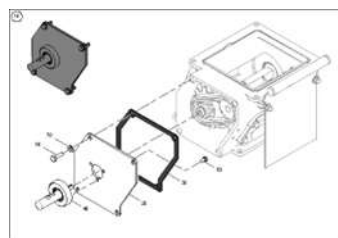
ЕТВ-0000009056, Подкомплект механического привода до 02.2021
