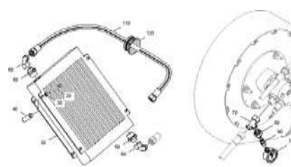
ETV-022514, Охлаждение масла / подогрев воздуха
