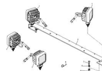
ЕТВ-022478, Светодиодное рабочее освещение 4 элем.
