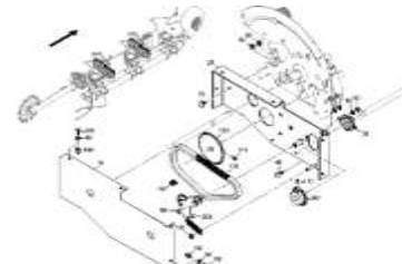
ЕТВ-0000001364, Приводные валы / подающая линия Citan мех.
