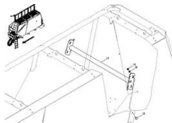
ЕТВ-0000004191, Бункер 7800L / распорка
