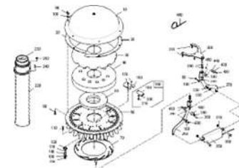
ЕТВ-022407, Распределительная головка с технологической колеей, 36 выпусков (12001-C)
