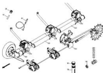
ЕТВ-0000010933, Конвейерная линия Citan механическая
