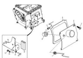
ЕТВ-022428, Одиарный дозатор пр. - комплект деталей системы подачи под давлением
