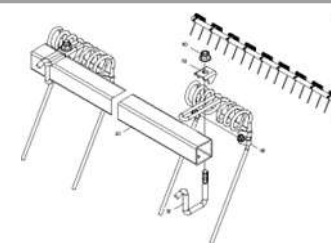
ЕТВ-0000004559, Балка бороны HD 3000 166
