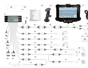
ETB-6000000177, 67600135 Базовый комплект электроники СКИФ-28 до 12.2025
