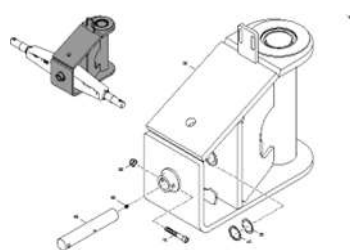
ETB-0000004185, Базовая машина Citan 12001-C, 15001- С дышло
