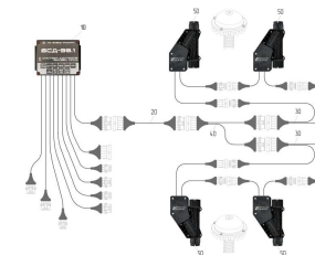
ETB-6000000201, 67600471 Технологическая коlea с клапанами с СКИФ-28 в базе (опция) до 02.2026
