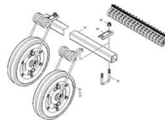
ЕТВ-0000004566, Катковая балка 330 3000 166
