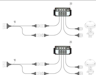
ЕТВ-6000000200, 67600472 Технологическая колея с актуаторами с СКИФ-38 в базе (опция) с 02.2026
