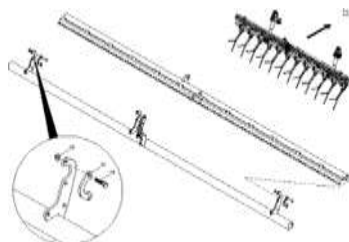
ЕТВ-0000001034, Основная труба выравнивателя 3000 С (02/K5)
