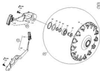
ETB-0000004689, Каток для ограничения глубины Control 25 с выступами сошник RoTeC pro с 02.2019
