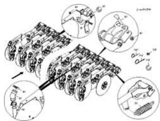
ЕТВ-0000004679, Комплект сошников Citan 12001 из 72 сошников RoTeC pro / pro-S (2)
