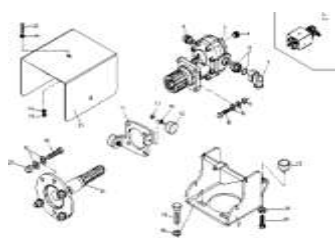
ETV-022511, Гидравлические детали подвижного насоса K700 35CCM
