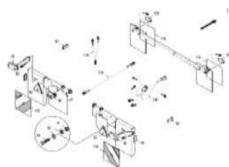
ETB-0000004337, Освещение CN 1 (3)
