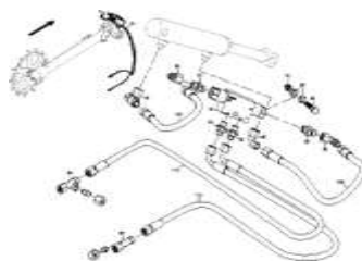
ЕТВ-0000001369, Колесо с почвозацепами гидравлические детали
