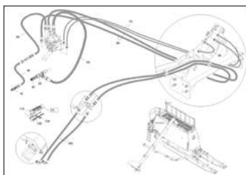
ETB-0000004471, Загрузочный шнек Citan Condor / MBG гидравлика шланги
