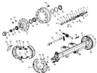
ЕТВ-022485, Тормозная ось, отдельные детали LA162
