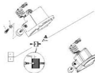
ЕТВ-022495, Радарный датчик международный / UK
