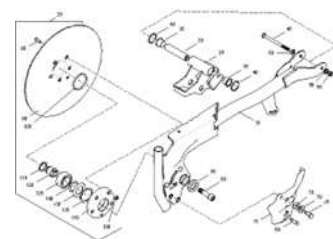
ЕТВ-022435, RoTeC Pro MI S длинный
