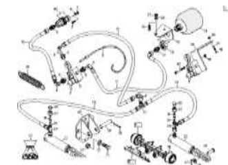
ЕТВ-022491, Ось с гидравлической тормозной системой
