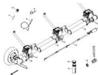
ETB-0000010911, Конвейерная линия Citan, электрическая
