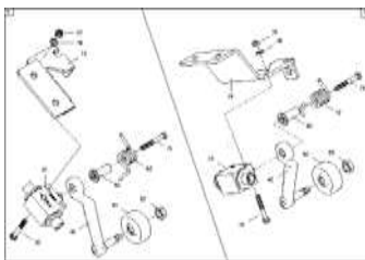
ЕТВ-022509, Переключающий клапан устройства складывания Citan 12001
