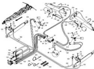
ЕТВ-022508, Гидр. детали рама Citan 15001
