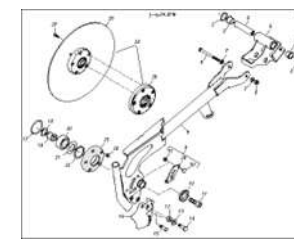
ЕТВ-0000004266, Сошник RoTeC pro длинный (221426) с 4.2019
