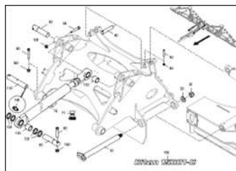
ЕТВ-0000004237, Задний модуль Citan 15001-C, задняя рама навесные детали
