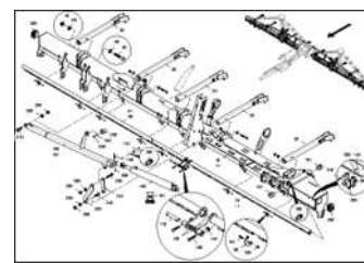
ЕТВ-0000004242, Задний модуль Citan 15001-C, консоль справа, слева (1)
