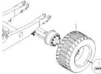
ЕТВ-022486, Комплект колес 700/50-26,5
