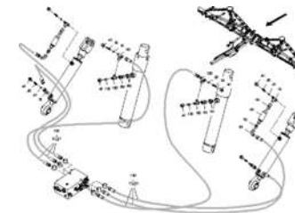
ЕТВ-0000004273, Задний модуль Citan 15001-C, гидр. детали консоль
