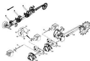
ЕТВ-0000010976, Конвейерная линия Citan механическая, приводная
