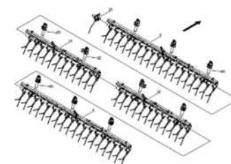
ETB-022457, Выравниватель Exakt S 15000
