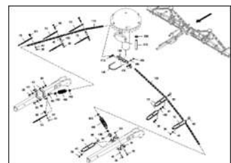
ЕТВ-0000004249, Задний модуль Citan 15001-C, консоль слева, справа (3)
