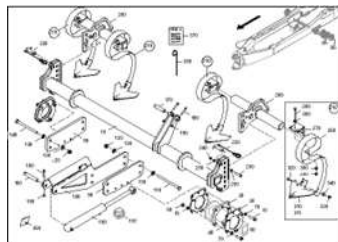
ЕТВ-0000006699, Стабилизатор колес трактора
