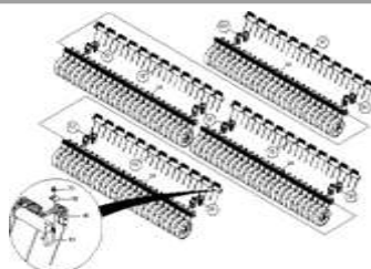
ЕТВ-0000004640, Каток выравниватель 330 12000 125 4Т
