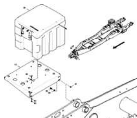
ETB-0000004177, Базовая машина Citan 12001-C, 15001- отсек для хранения
