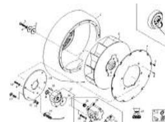
ETB-022410, Подающая линия 12001-15001-C вентилятор
