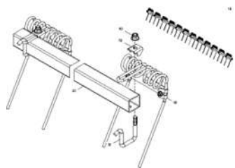
ЕТВ-0000004649, Балка бороны HD 3000 125
