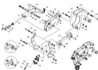
ЕТВ-0000004500, Крепление катка-выравнивателя CIT01 предв. смонт.
