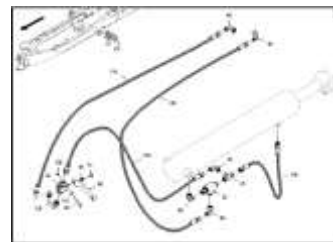
ЕТВ-0000006700, Гидравлические детали колесного молота трактора
