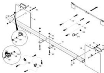
ETB-0000004332, Освещение CN 1 (2)
