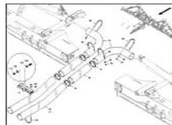
ЕТВ-0000004204, Задний модуль Citan 12001-C 15001-C, подающая труба
