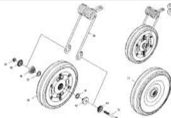
ЕТВ-0000004660, Каток 330x65 с пружиной
