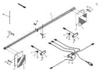
ETB-022479, Освещение для движения по дороге Citan 12001-C / 15001-C (1)
