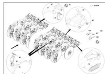
ЕТВ-0000004683, Комплект сошников Citan 15001 из 90 сошников RoTeC pro / pro-S (2)
