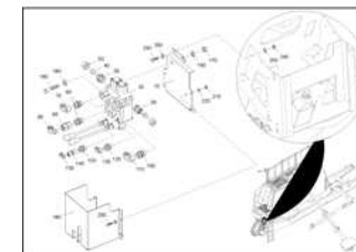
ETB-0000004470, Загрузочный шнек Citan Condor / MBG блок управления гидравлики
