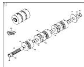
ЕТВ-0000007799, Дозирующий ролик 20 см³
