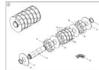
ЕТВ-0000007900, Дозирующий ролик 210 см³
