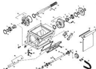
ETB-022418, Однократное дозирование 2.0 Привод вправо
