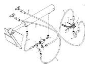
ЕТВ-022502, Гидр. детали рыхлитель колеи трактора
