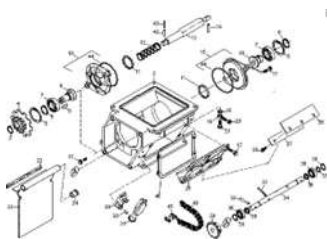
ETB-022417, Однократное дозирование 2.0 Привод слева
