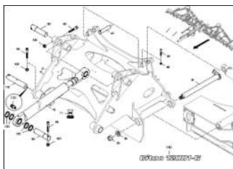
ЕТВ-0000004199, Задний модуль Citan 12001-C, задняя рама навесные детали
