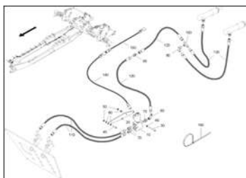
ЕТВ-0000007000, Гидравлические части маркеров технологической колеи Citan
