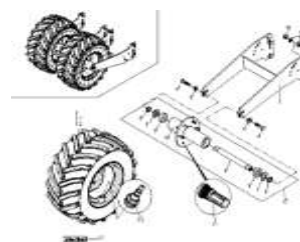
ETB-022455, Комплект копирующих колес до 02.2020
