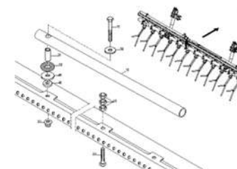
ЕТВ-0000001068, Регулировочный рычаг
