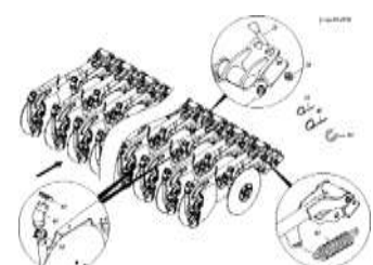
ETV-0000004667, Комплект сошников Citan 12001 из 96 сошников RoTeC pro / pro-S (2)
