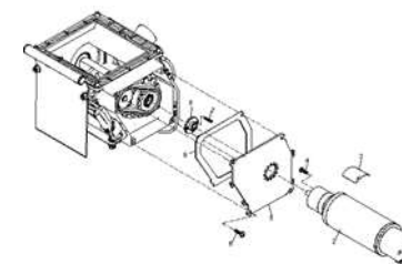
ЕТВ-022427, Одиарный дозатор пр. - комплект деталей эл. привод
