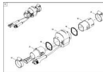
ETB-0000008898, Датчик контроля посевной линии Slue
