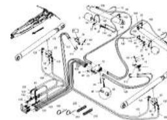
ЕТВ-022507, Гидр. детали рама 12001
