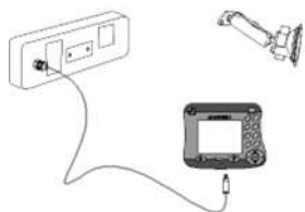
ЕТВ-022518, Внешняя световая балка для AmaTron 3
