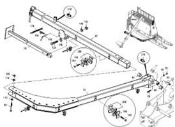
ETB-0000004466, Загрузочный шнек Citan Condor / MBG кронштейн
