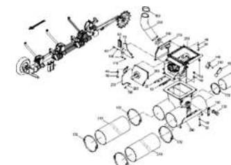
ЕТВ-0000010975, Конвейерная линия Citan, механическая (3)
