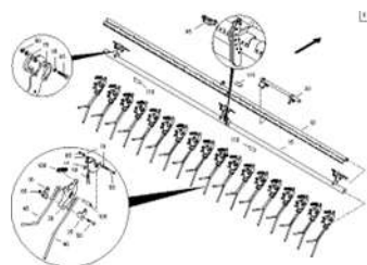
ЕТВ-022458, Выравниватель Exakt 4500 S 15000 - отдельные детали
