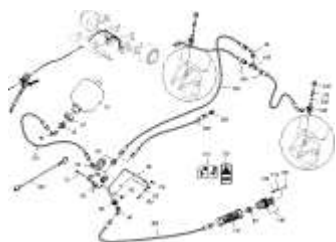
ЕТВ-0000006553, Мост с гидравлической тормозной системой 12001-С/15001-С 8000L (2)
