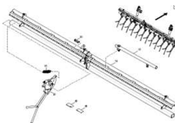
ETB-0000001035, Выравниватель Exakt 3000 125 15 C
