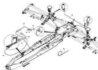
ЕТВ-0000006178, Кабельный комплект Digitroll распределительная головка 2
