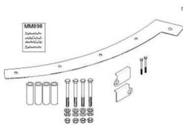
ETB-0000004472, Комплект дооснащения загрузочный шнек Citan / Condor
