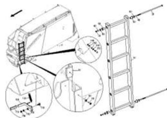
ЕТВ-0000004193, Бункер 7800L / лестница
