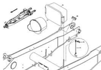
ETB-0000004176, Базовая машина Citan 12001-C, 15001- С навесные детали
